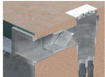
Pormenor de instalação do skimmer
