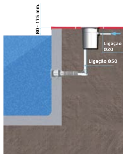
Pormenor de instalação do regulador de nível
