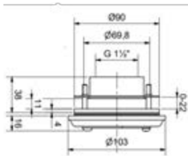
Dimensões da boca de aspiração com tampa AISI 316L
