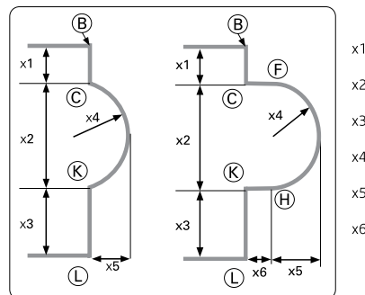
Escada Romana (raio constante) Dimensões (em m)
