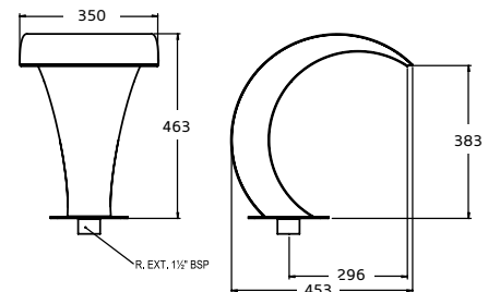
B - Cascata residencial onda (AISI 316L)
