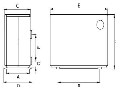
Dimensões bomba de calor FULL INVERTER - Mr. Silence
