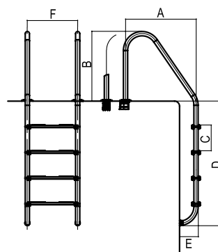
A - Escada standard inox inclui ancoragem com ligação terra (AISI 316L)
