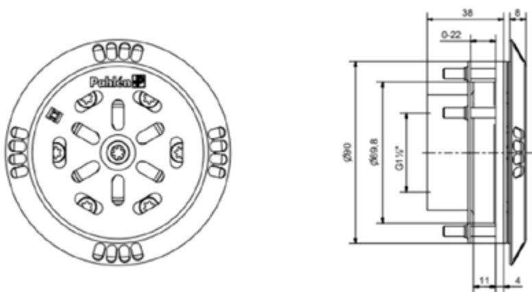
Dimensões boca de impulsão de fundo AISI 316L
