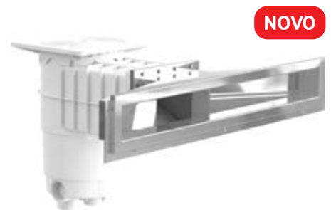
A - Skimmer ABS + AISI 316L (liner / betão) - Design A800i (806 x 126 mm)
