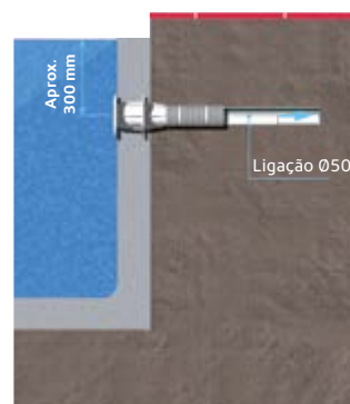
Pormenor de instalação da boca de aspiração.
