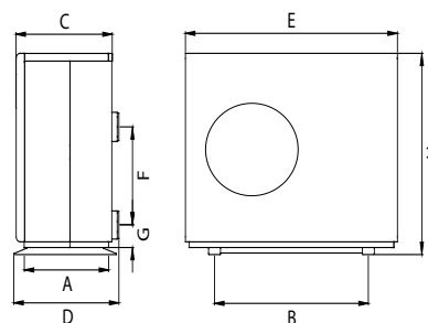
Dimensões bomba de calor FULL INVERTER - Série Mr. Smile
