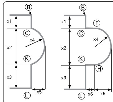
Escada Romana (raio constante) Dimensões (em m)
