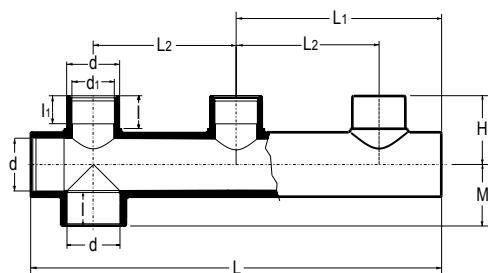
B - Coletor com saída lateral
