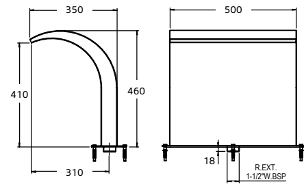
A - Cascata residencial A (AISI 316L)
