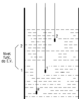
Esquema do posicionamento das 3 sondas
