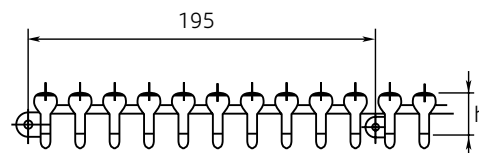
A - Placa grelha transversal
