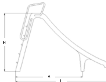
D - Escorrega Pranaslide
