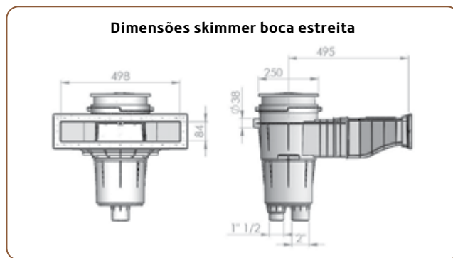
A - Skimmer ABS tampa quadrada - boca estreita - Branco
