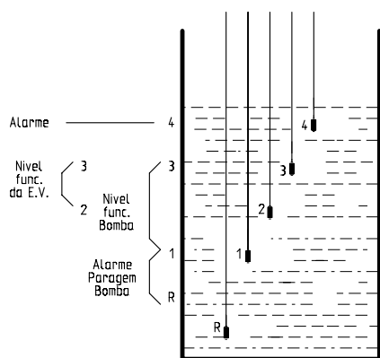
Esquema do posicionamento das 5 sondas
