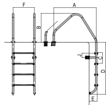
A - Escada para piscina com caleira inclui ancoragem com ligação terra (AISI 316L)
