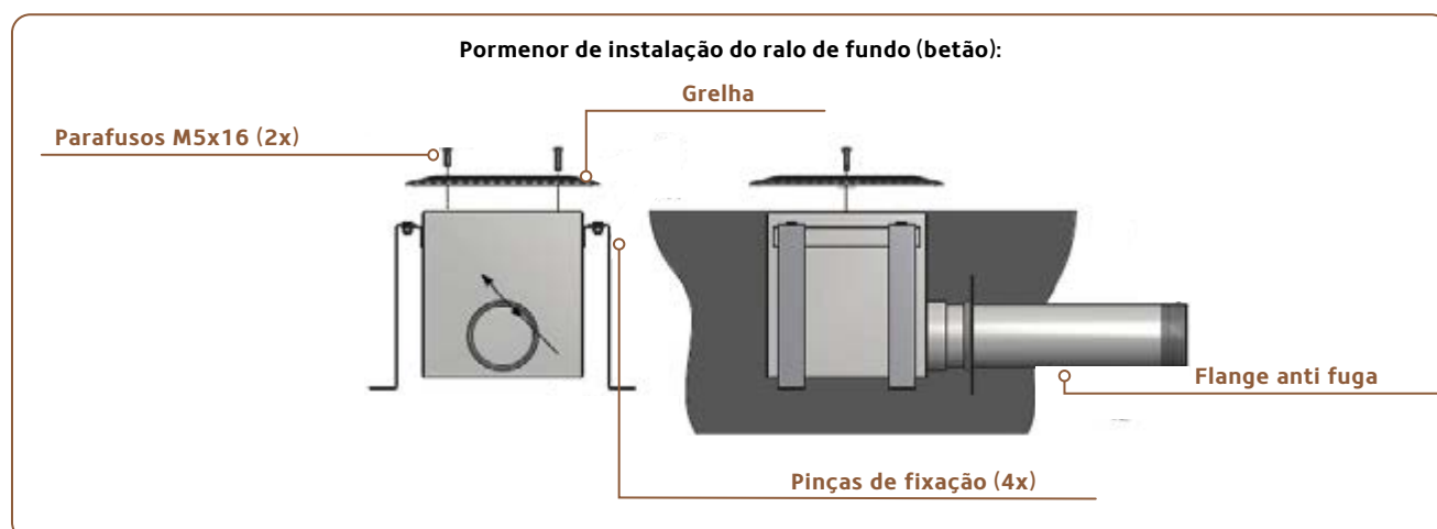
A - Ralo de fundo AISI 316L retangular 191 x 181 mm (betão) - saída lateral 2"
