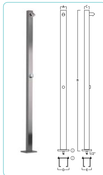
A - Chuveiro inox Deluxe Light (AISI 316L)
