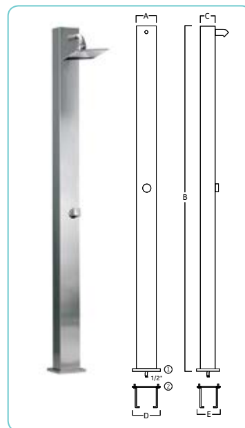
B - Chuveiro inox Deluxe Light Pro (AISI 316L)
