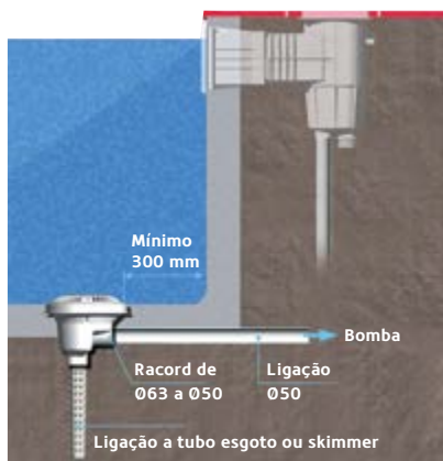
Pormenor de instalação do ralo de fundo
