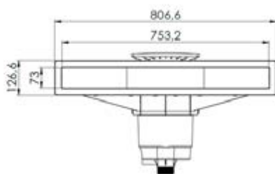
Dimensões da versão com revestimento de betão
