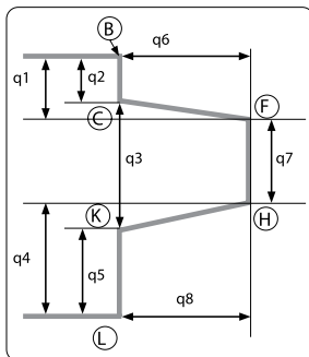
Escada Trapézio Dimensões (em m)
