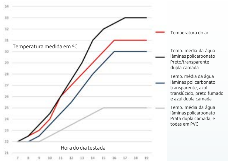
Comparativo de poder de aquecimento segundo o modelo das lâminas
